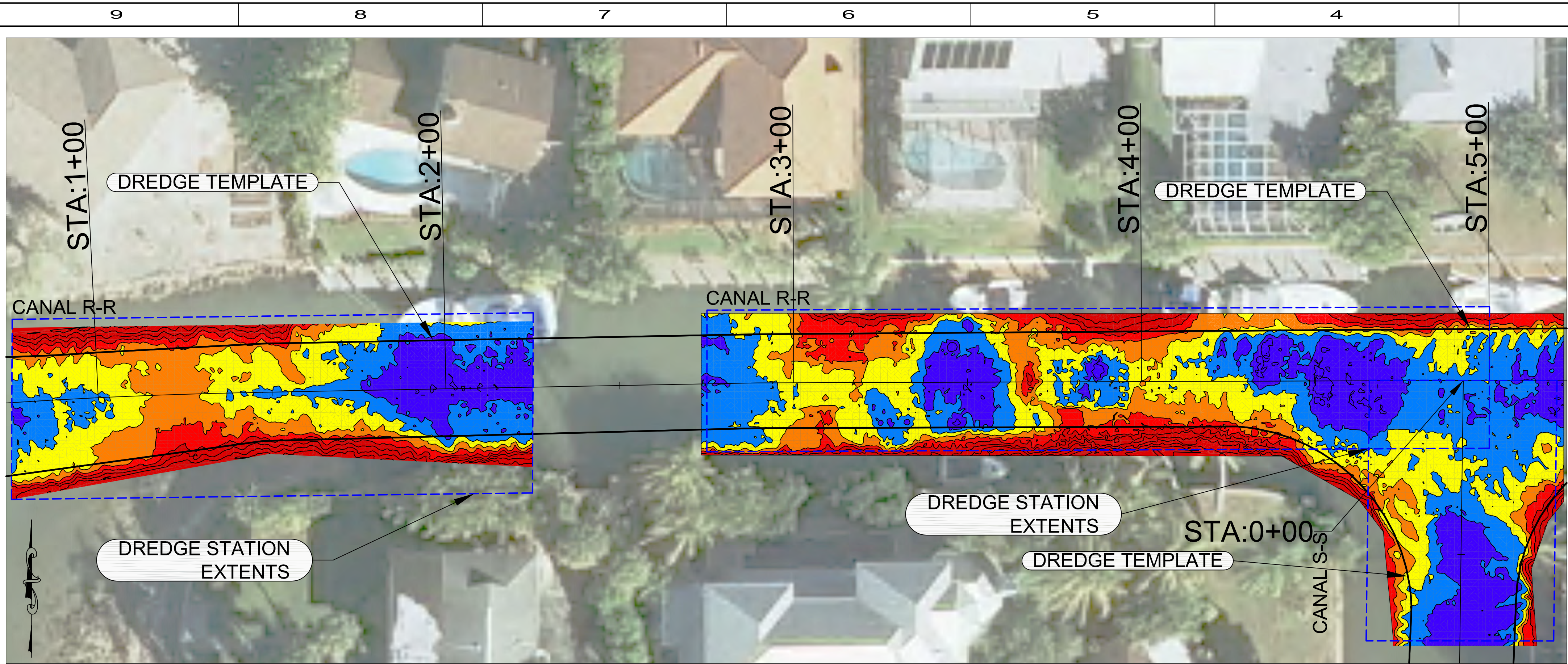
DREDGE EXTENTS R-R STA. 0+75 TO STA. 2+25 AND STA. 2+75 TO STA. 5+00
