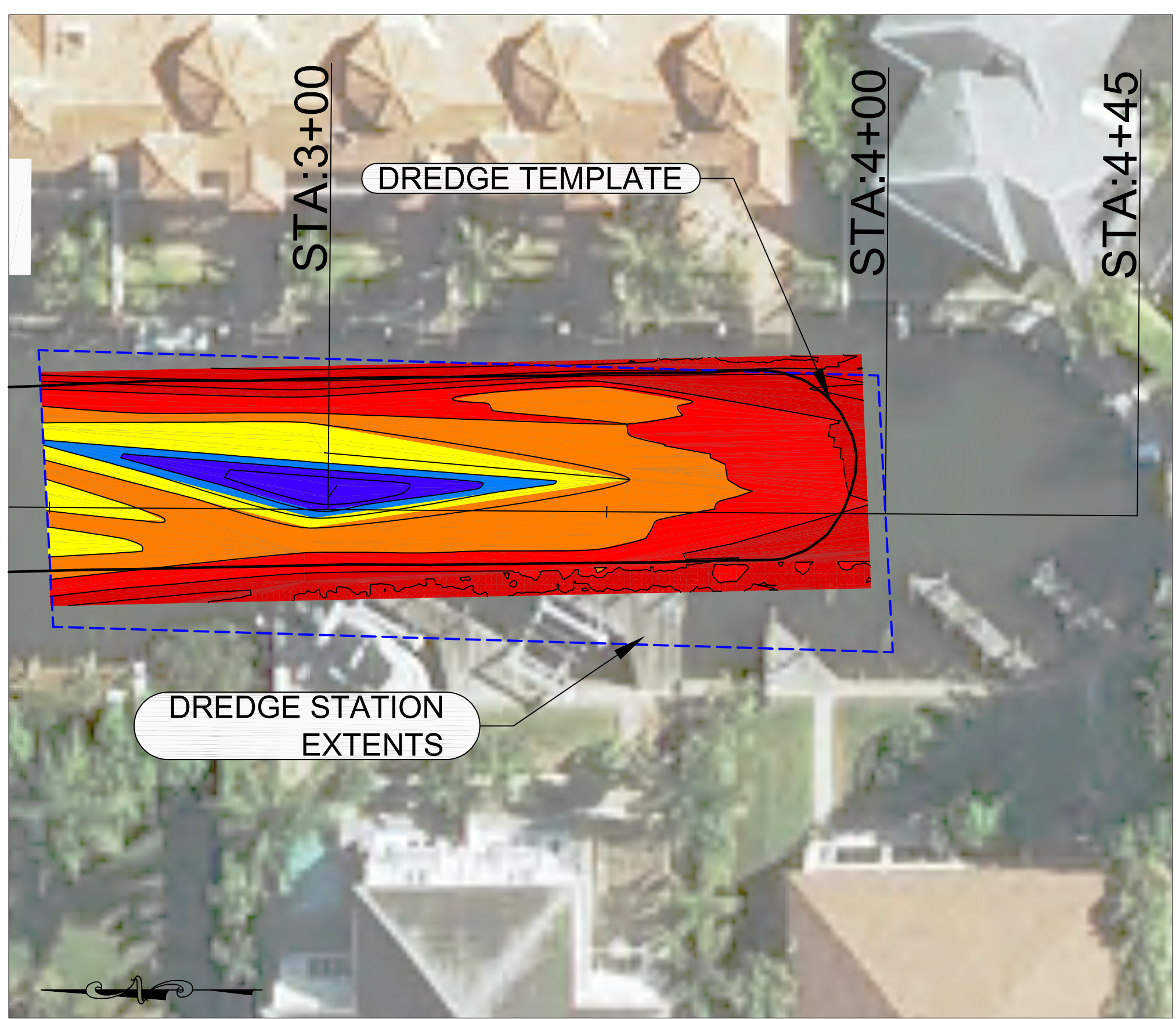
DREDGE EXTENTS Y-Y STA. 2+50 TO STA. 4+45
