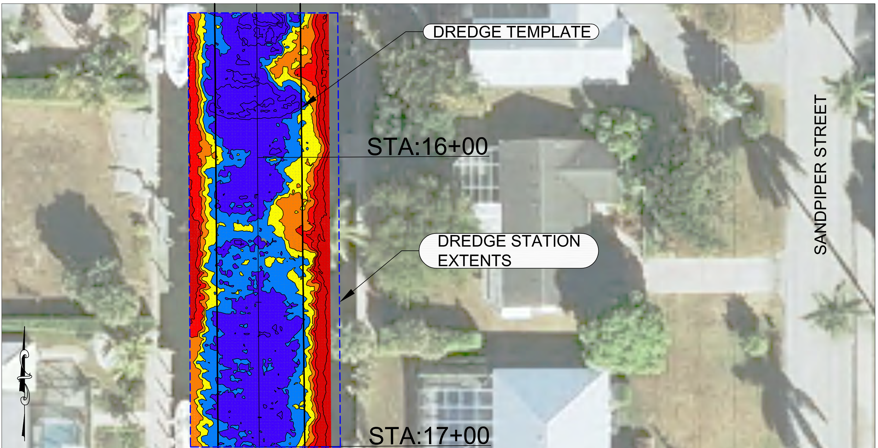
DREDGE EXTENTS R-R STA. 15+50 TO STA. 17+00
