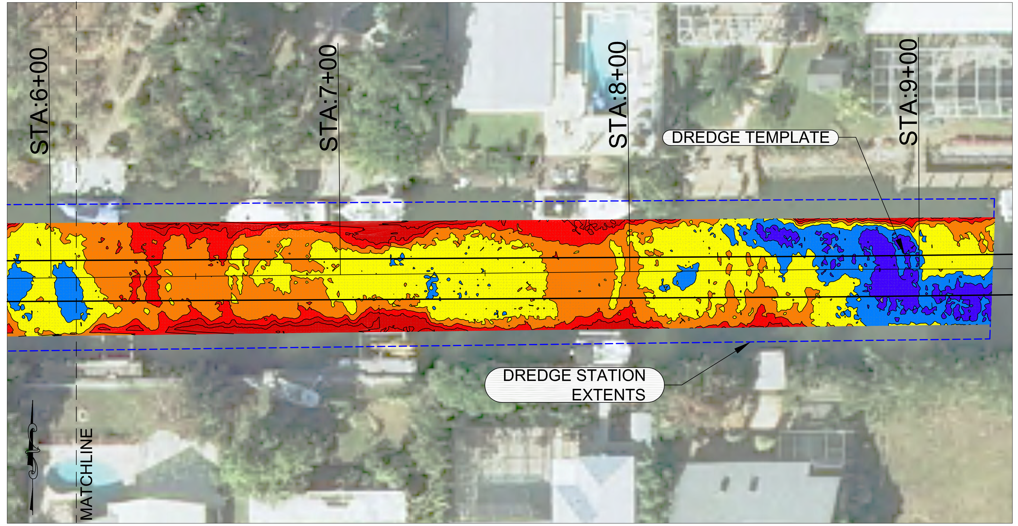
DREDGE EXTENTS BB-BB STA. 2+75 TO STA. 9+25
