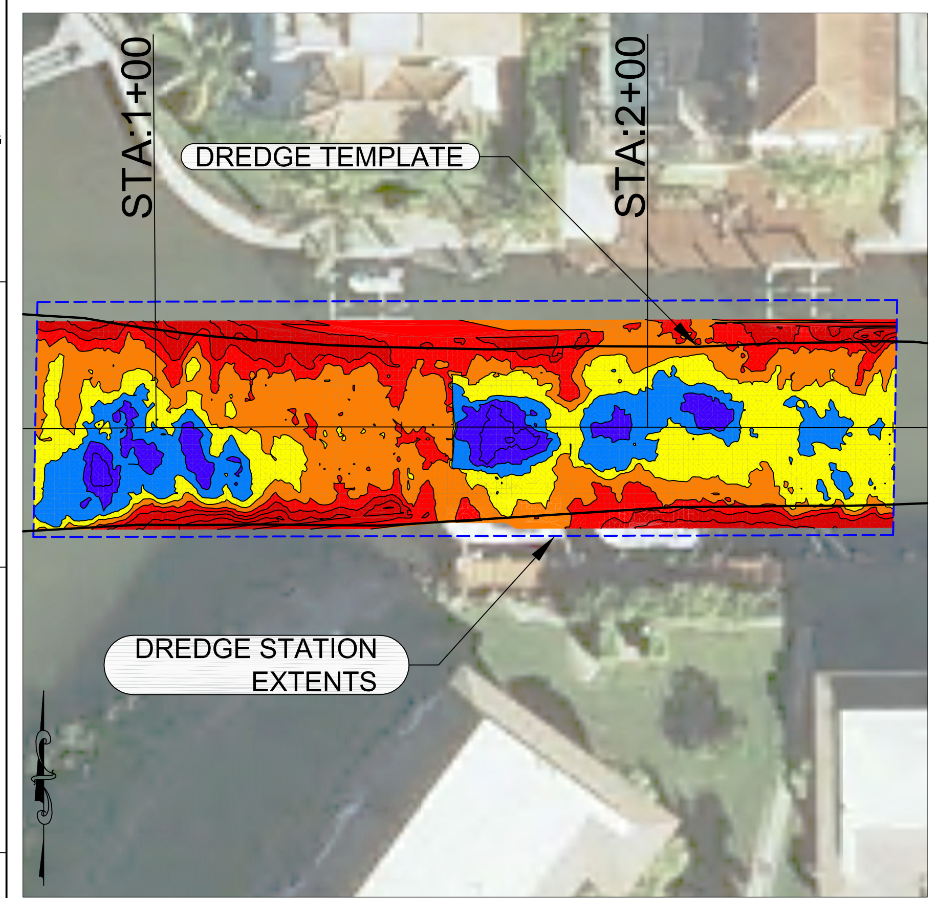
DREDGE EXTENTS X-X STA. 0+75 TO STA. 2+50
