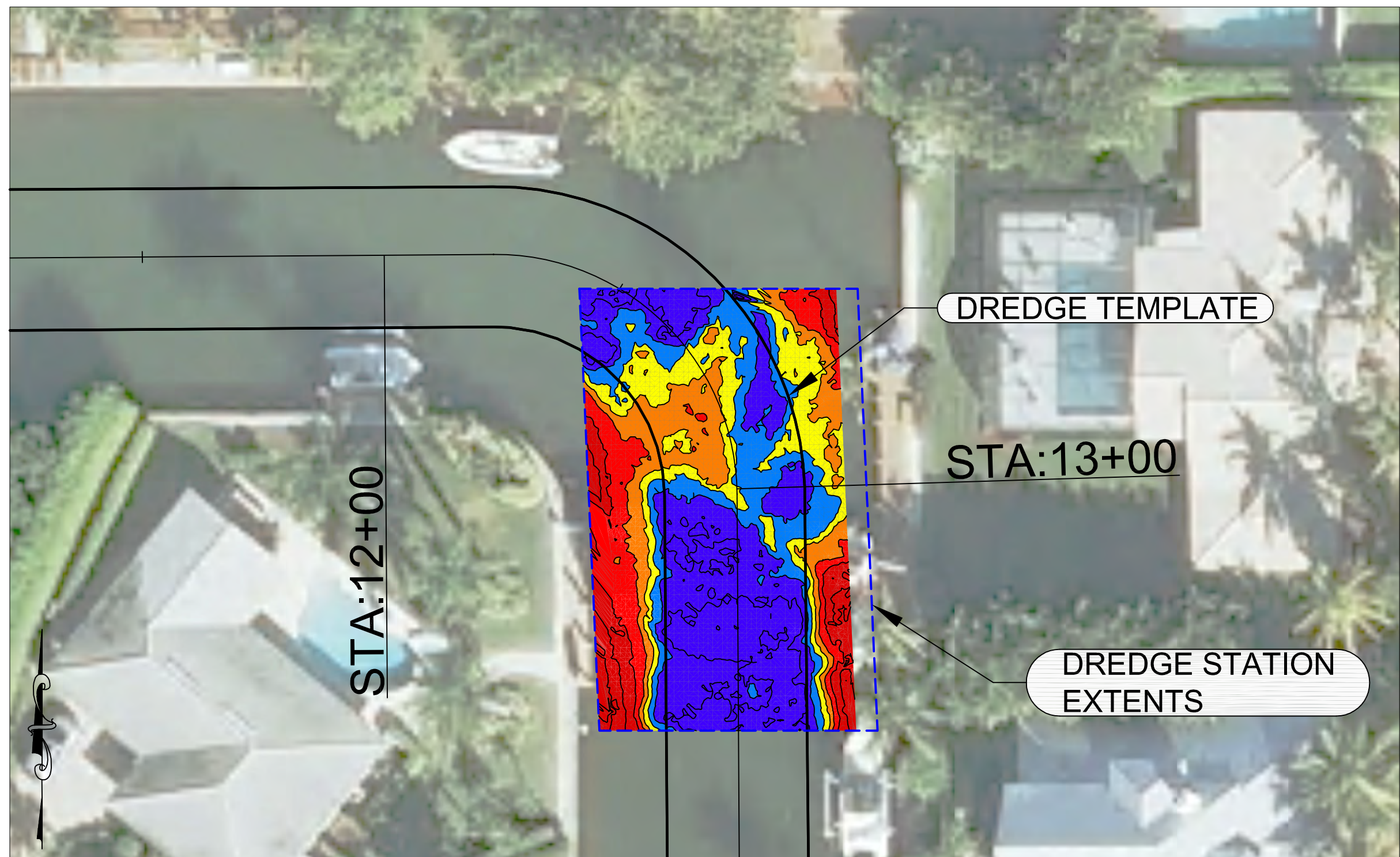
DREDGE EXTENTS R-R STA. 12+50 TO STA. 13+50
