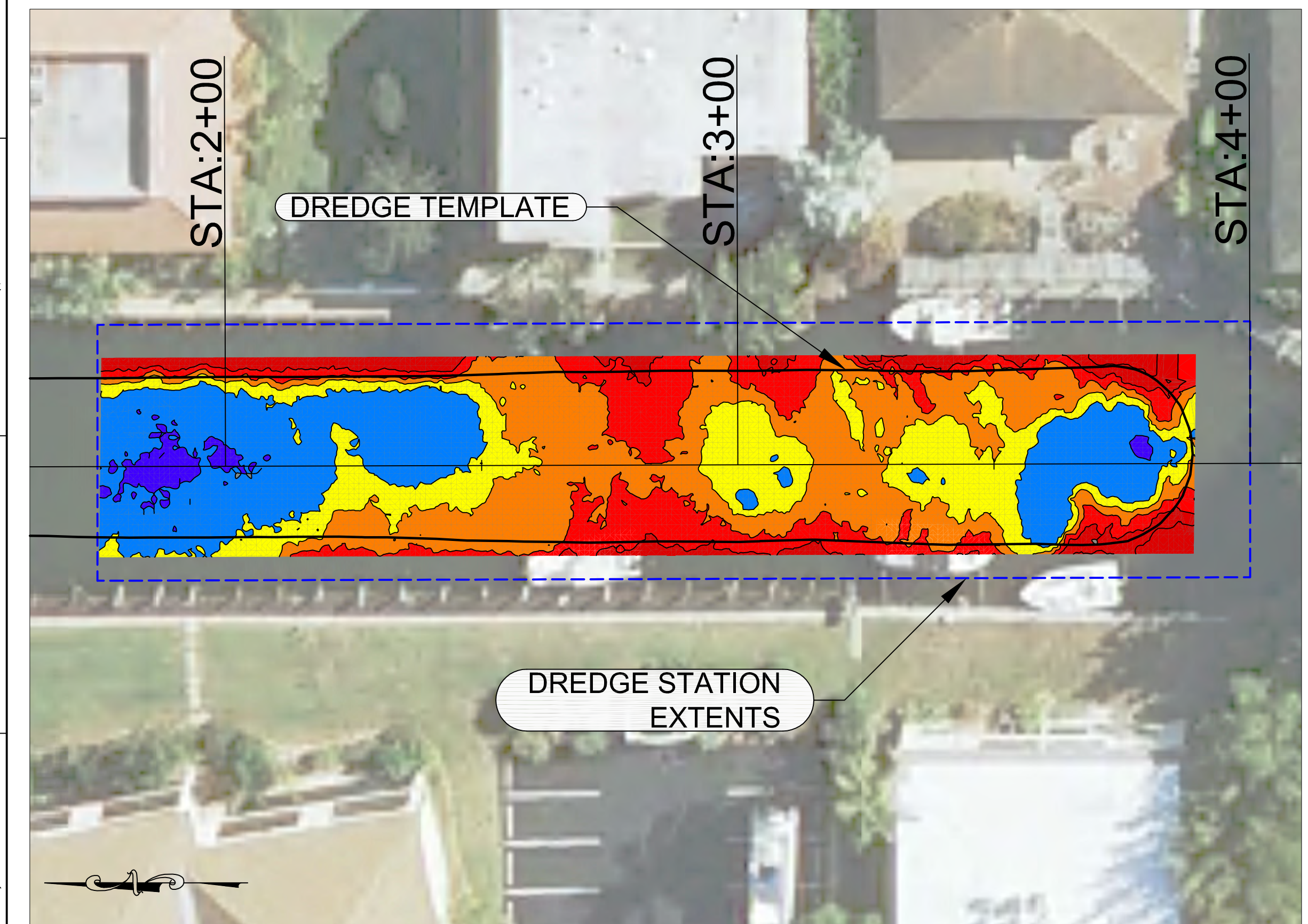
DREDGE EXTENTS Z-Z STA. 1+75 TO STA. 4+00
