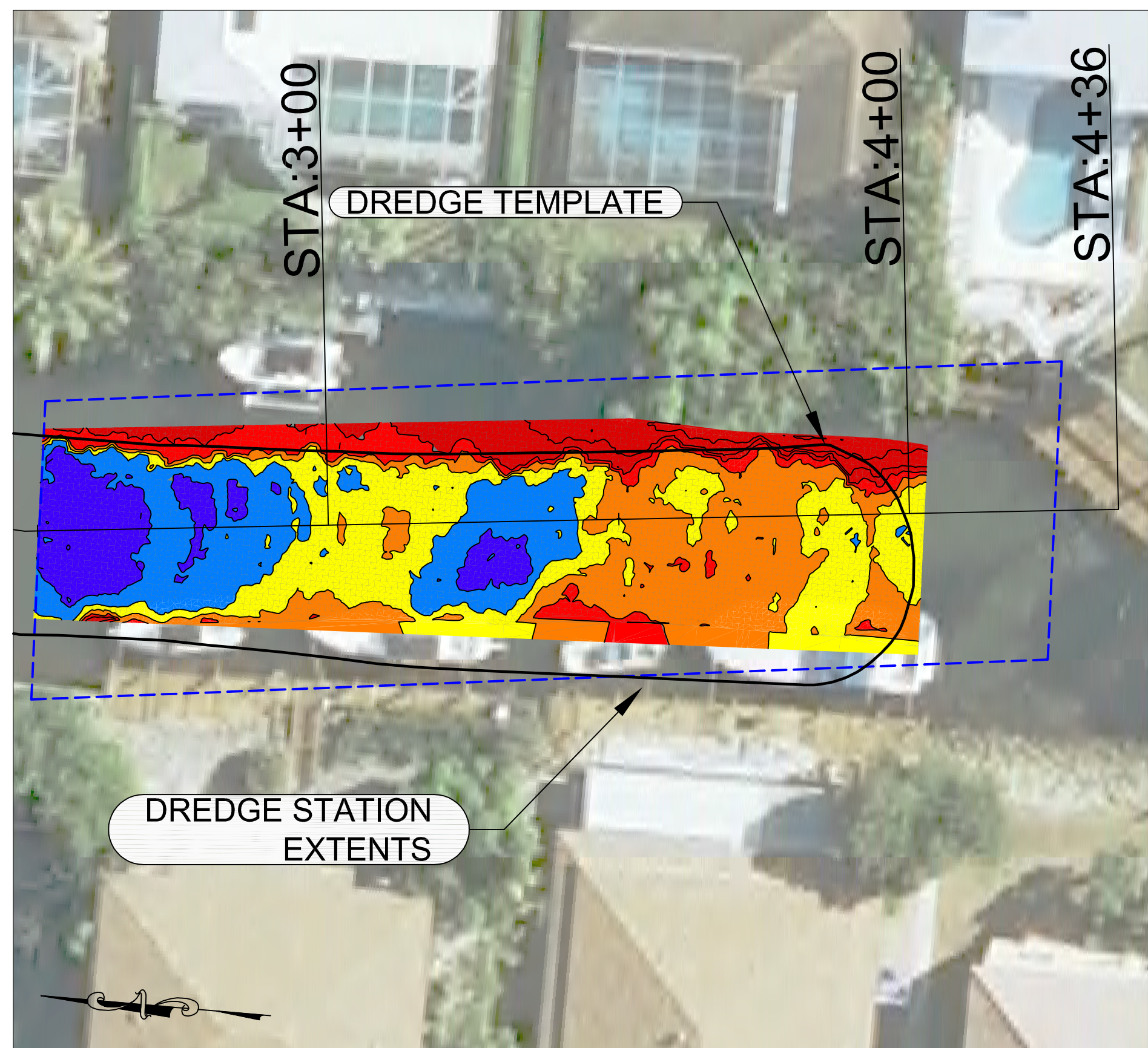
DREDGE EXTENTS AA-AA STA. 2+50 TO STA. 4+36
