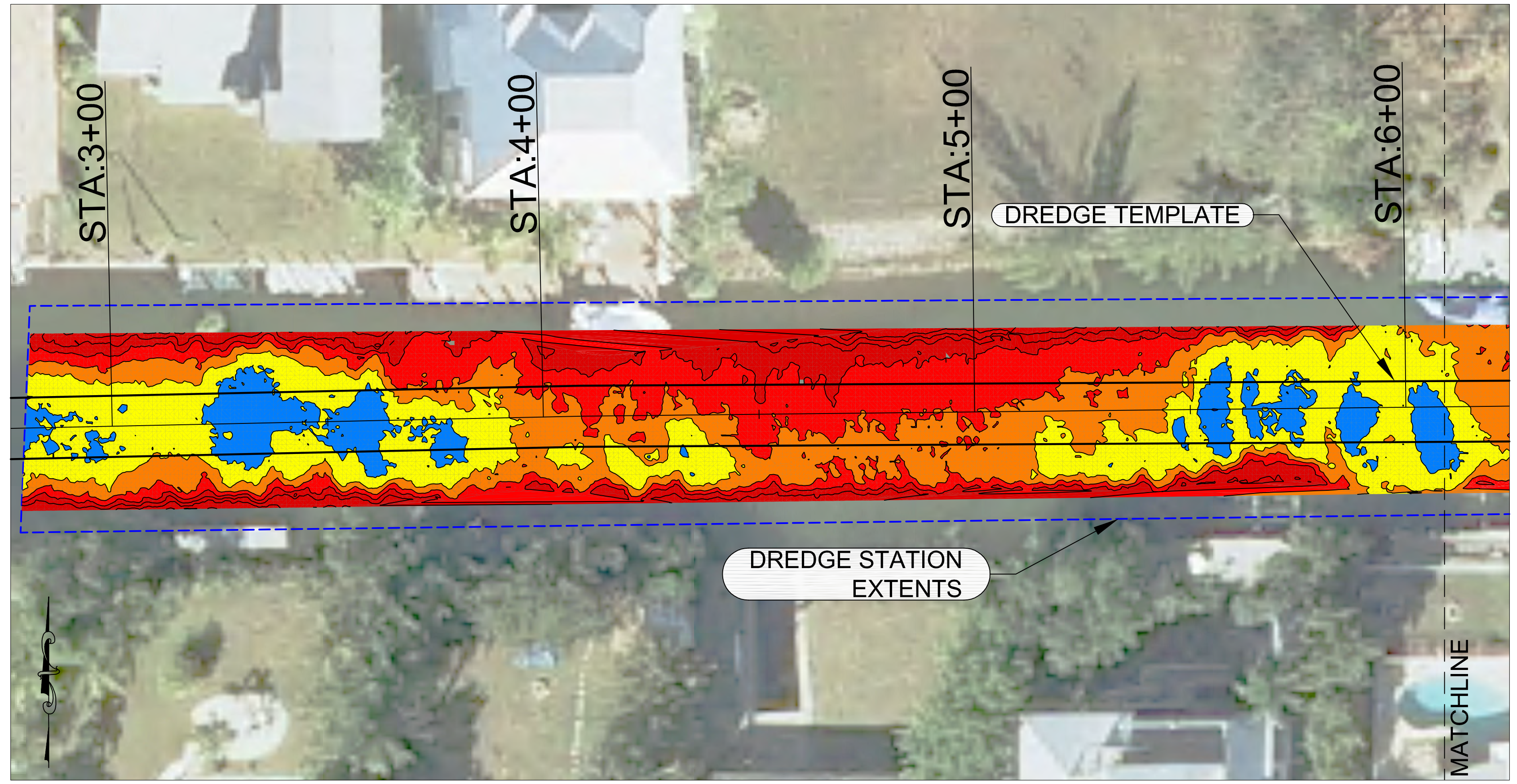
DREDGE EXTENTS BB-BB STA. 2+75 TO STA. 9+25
